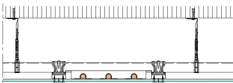
Schnitt geschlossene GK-Decke
