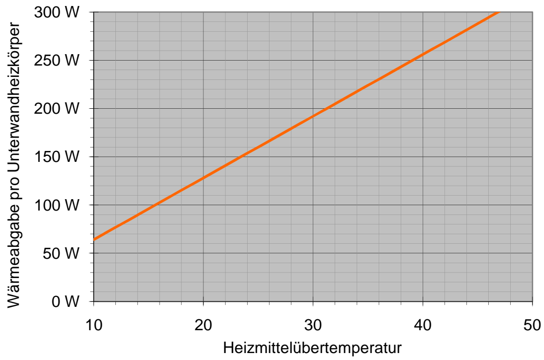
Leistungsdiagramm cupronova R6
