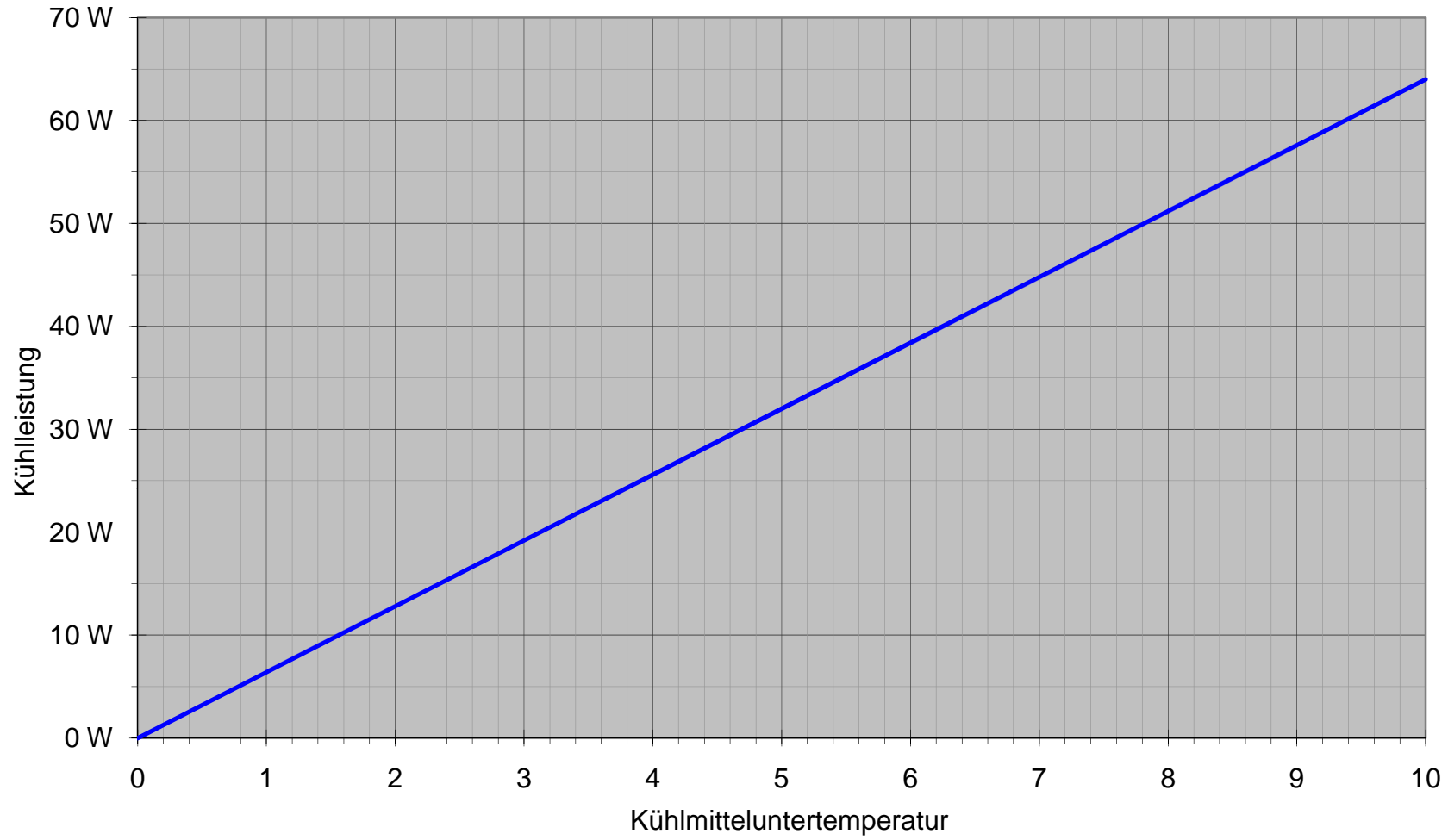
Kühlen - Leistungsdiagramm cupronova
